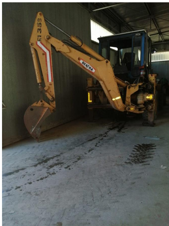
Foto 3 Terna Meccanica, Marca BENFRA Mod. 1.35B
